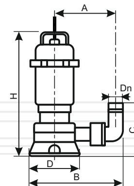
Габаритні та приєднувальні розміри
