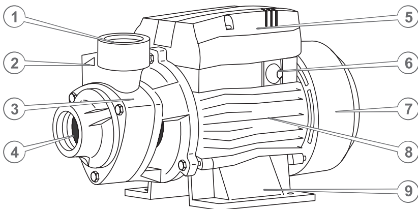
Рисунок 2. Зовнішній вигляд насосів групи моделей «PQ».
