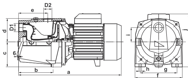
Рисунок 12. Габаритні та приєднувальні розміри насосів групи моделей «JW».
