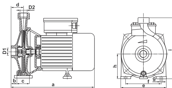
Рисунок 6. Габаритні та приєднувальні заміри насосів групи моделей «CP» (таблиця 2).
