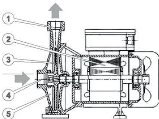
Рисунок 4. Схема конструкції насосів поверхневих групи моделей «CP» (фронтальний перетин).
