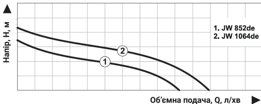
Рисунок 17. Форма діаграми напірно-витратної характеристики насосів поверхневих моделі «JW 1064de».
