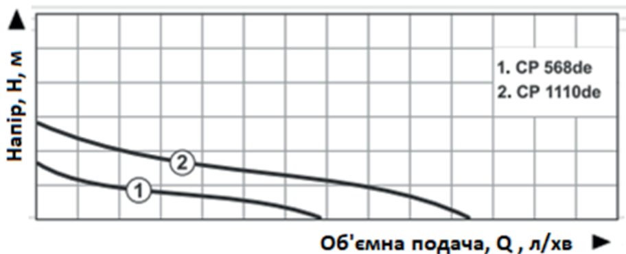
Рисунок 15. Форма графіка напірно-витратної характеристики насосів поверхневих моделей «CP 568de» та «CP 1110de».
