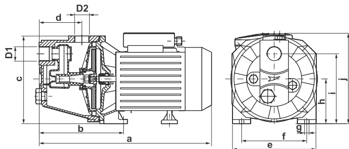
Рисунок 11. Габаритні та приєднувальні розміри насосів групи моделей «J».
