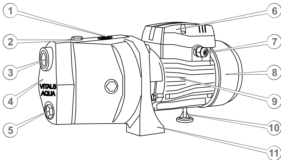
Рисунок 9. Зовнішній вигляд насосів групи моделей «JW».
