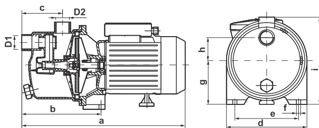
Рисунок 13. Габаритні та приєднувальні розміри насосів групи моделей «JS».
