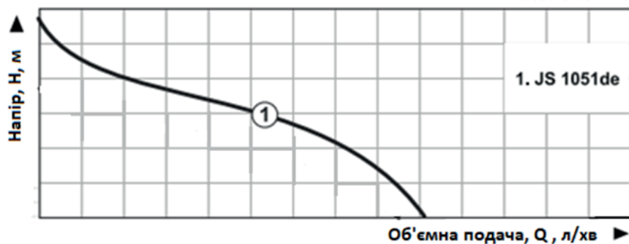
Рисунок 18. Форма графіка напірно-витратної характеристики насосів поверхневих моделі «JS 1051de».
