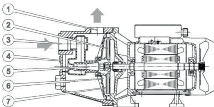
Рисунок 7. Схема конструкції насосів поверхневих групи моделей «J», «JW» та «JS» (фронтальний перетин).
