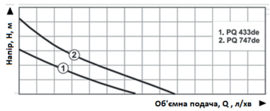
Рисунок 14. Форма графіка напірно-витратної характеристики насосів поверхневих моделей «PQ 433de» та «PQ 747de».
