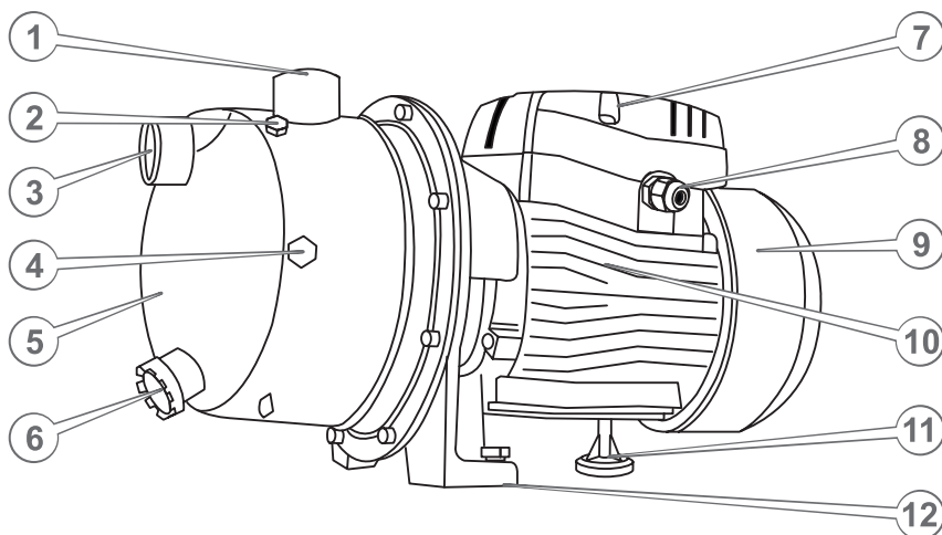
Рисунок 10. Зовнішній вигляд насосів групи моделей «JS».
