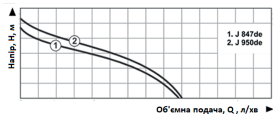
Рисунок 16. Форма графіка напірно-витратної характеристики насосів поверхневих моделей «J 847de» та «J 950de».
