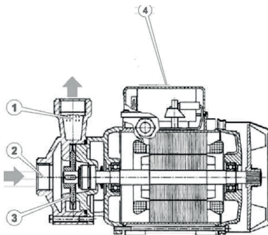
Рисунок 1. Схема конструкції насосів поверхневих групи моделей «PQ» (фронтальний перетин).
