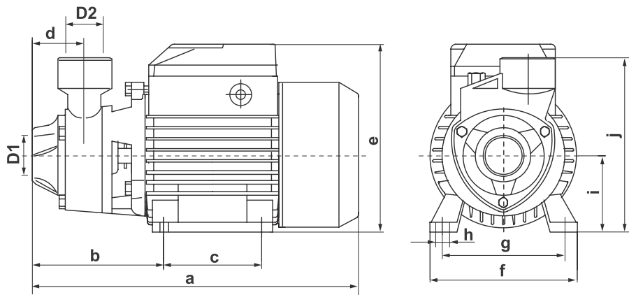
Рисунок 3. Габаритні та приєднувальні розміри насосів групи моделей «PQ» (таблиця 1).
