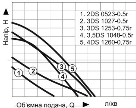
Рисунок 4. Форма діаграма напірно-витратної характеристики насосів занурювальних свердловинних шнекових моделей «2DS 0523-0.5r», «3DS 1027-0.5r», «3DS 1253-0.75r», «3.5DS 1048-0.5r», «4DS 1260-0.75r».
