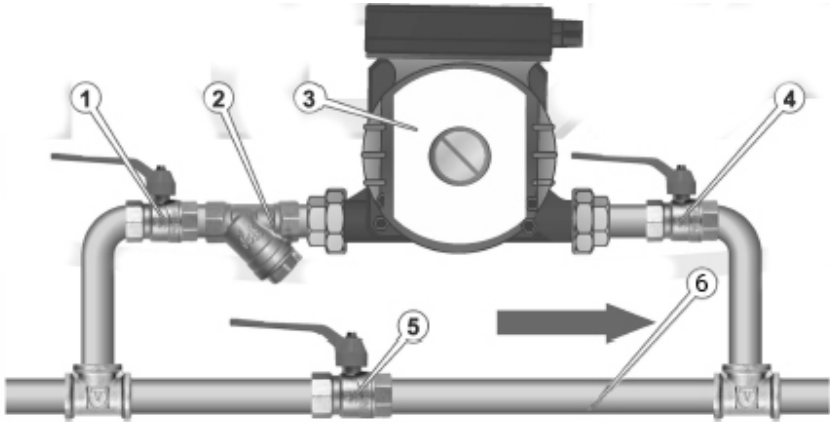
Рисунк 2. Схема встановлення насоса у систему.
