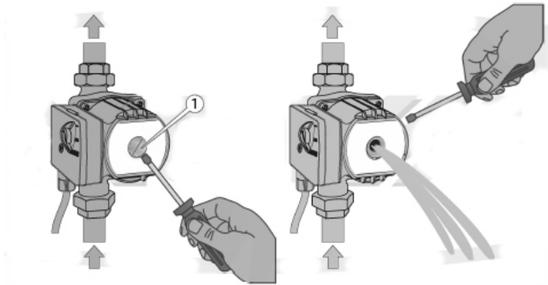
Рисунок 4. Схема випуску повітря з насоса.
